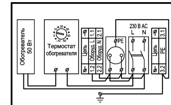
Рисунок 2 – Схема электрическая принципиальная
